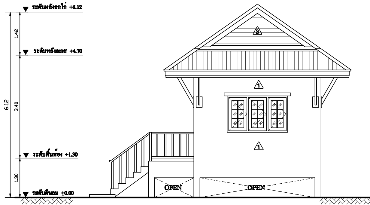
รูปด้าน 4 SCALE 1:75
