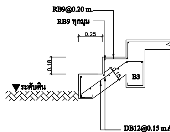
ST-2 SCALE 1:25
