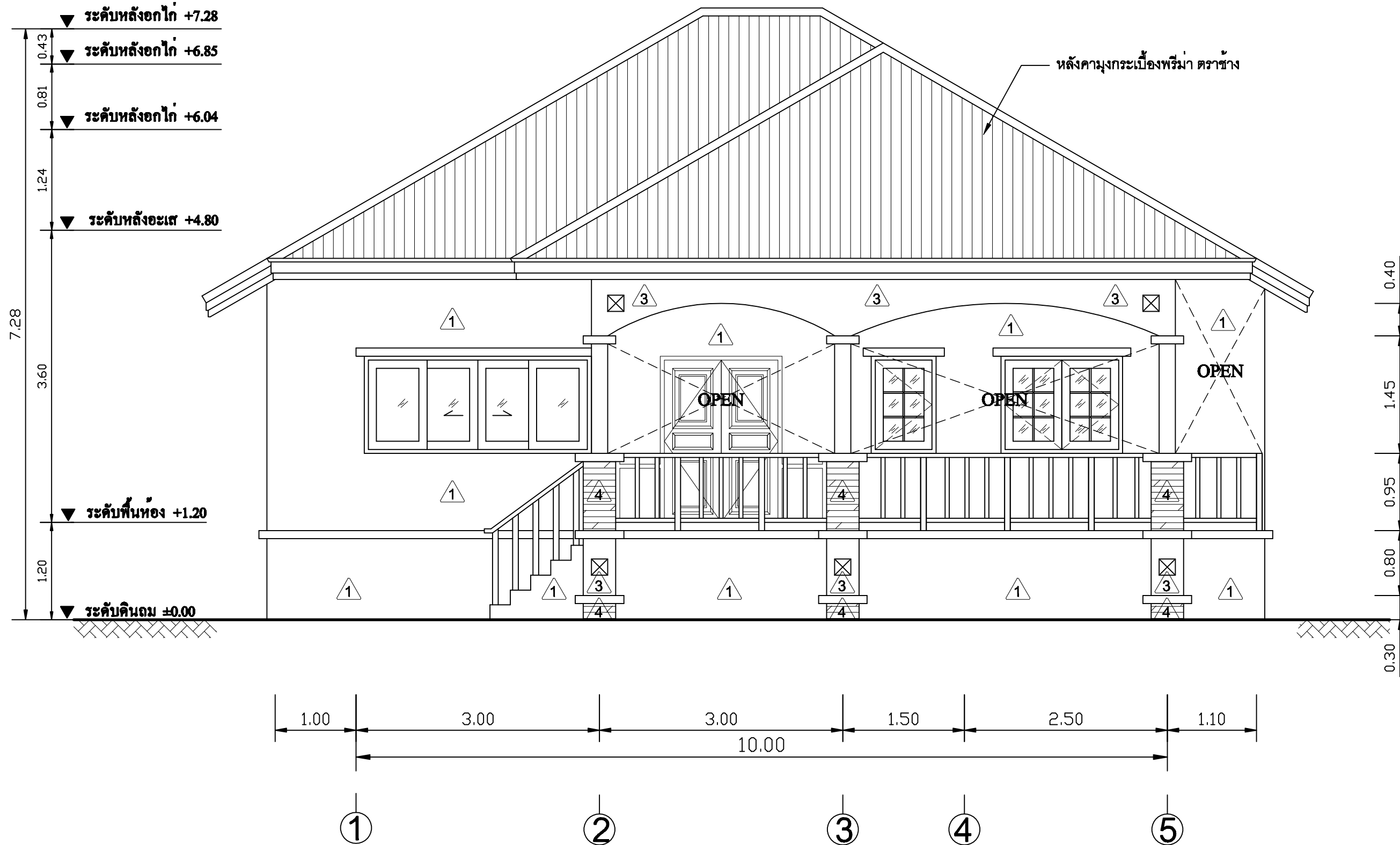
รูปด้าน 1 SCALE 1:50
