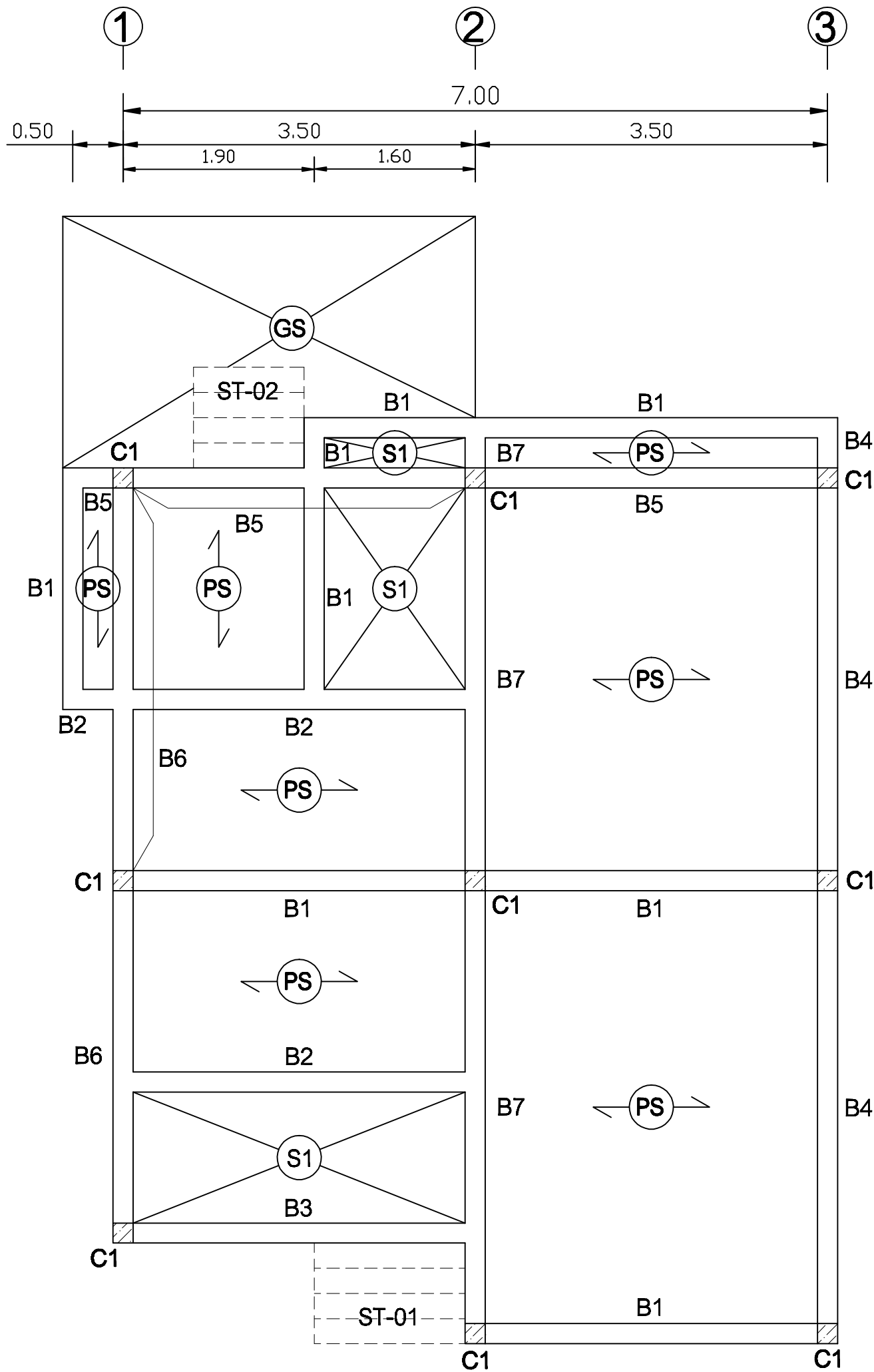
แบบโครงสร้าง SCALE 1:50
