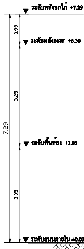
รูปด้าน 4 SCALE 1:75
