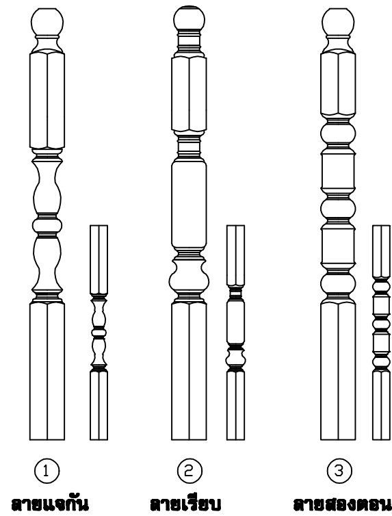
ลายลูกกรงบันได
