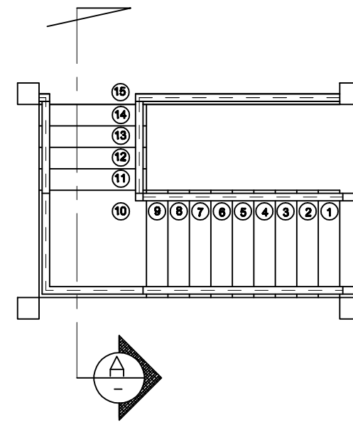
แปลนบันได SCALE 1:50
