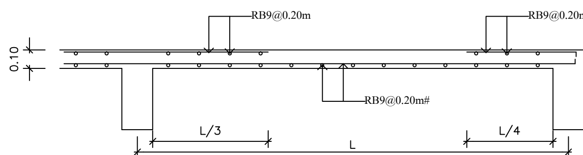
S1(ด้านยาว) SCALE 1:25
