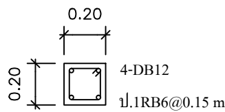
C1 SCALE 1:25
