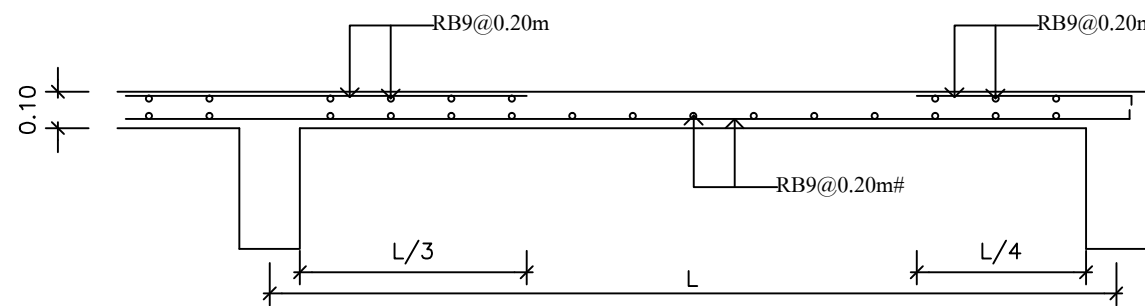
S1(ด้านสั้น) SCALE 1:25
