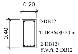
กลางช่วงคาน B1, RB1 SCALE 1:25
