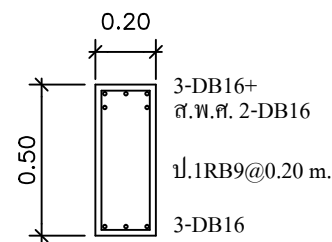
ช่วงเสา, คานขึ้น B5 SCALE 1:25
