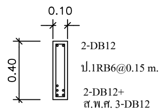
กลางช่วงคาน RB2 SCALE 1:25
