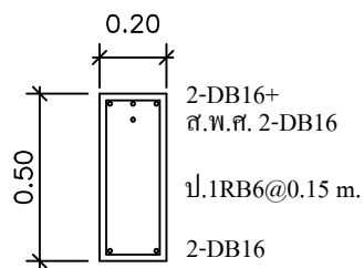
ช่วงเสา, คานขึ้น B4 SCALE 1:25
