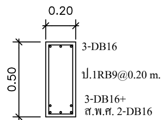
กลางช่วงคาน B5 SCALE 1:25
