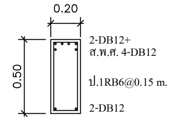
ช่วงเสา, คานขึ้น B3 SCALE 1:25
