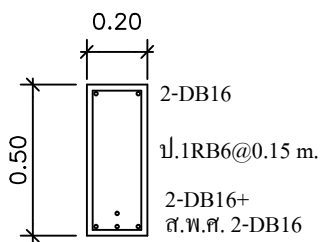
กลางช่วงคาน B4 SCALE 1:25
