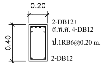
ช่วงเสา, คานขึ้น B2 SCALE 1:25
