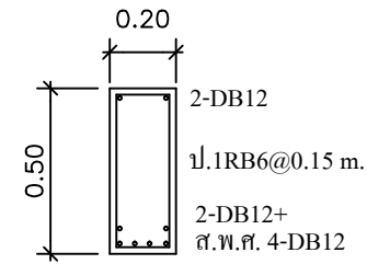
กลางช่วงคาน B3 SCALE 1:25
