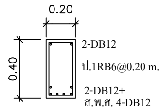
กลางช่วงคาน B2 SCALE 1:25
