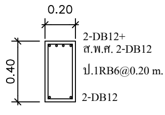
ช่วงเสา, คานขึ้น B1, RB1 SCALE 1:25
