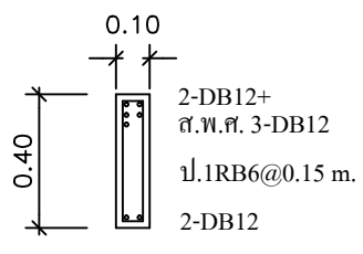
ช่วงเสา, คานขึ้น RB2 SCALE 1:25
