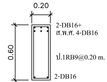
ช่วงเสา, คานขึ้น B6 SCALE 1:25
