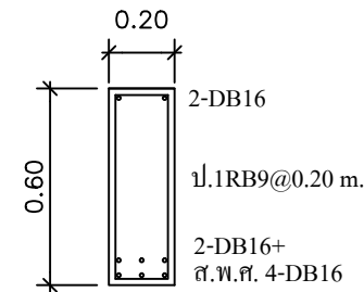
กลางช่วงคาน B6 SCALE 1:25
